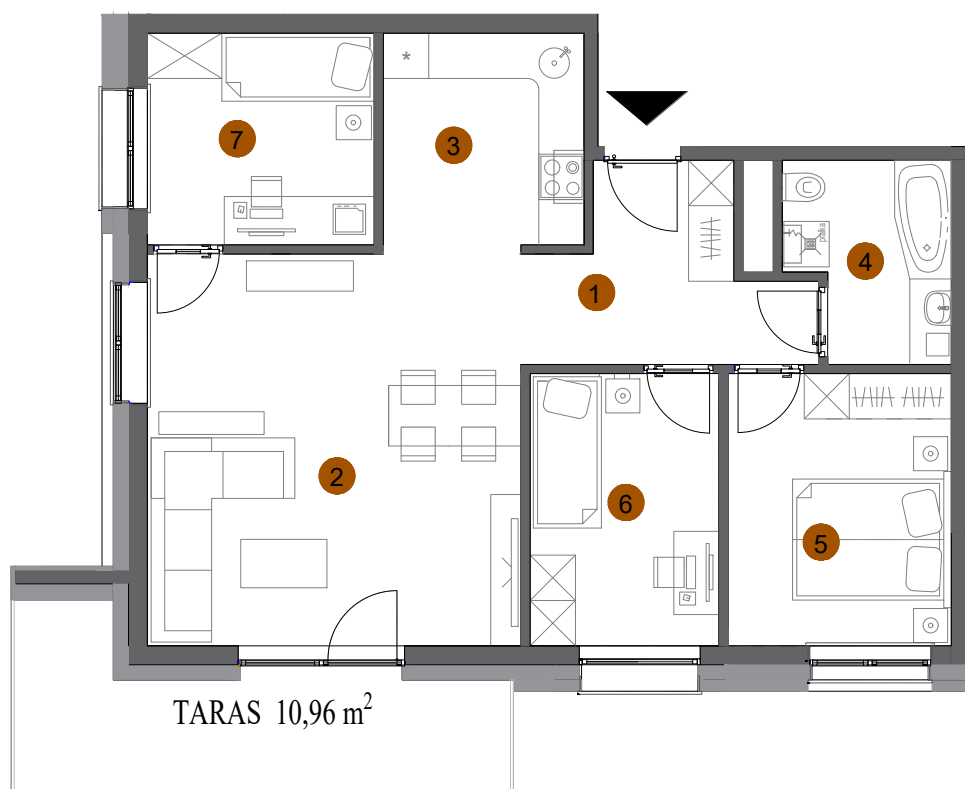
RZUT MIESZKANIA
