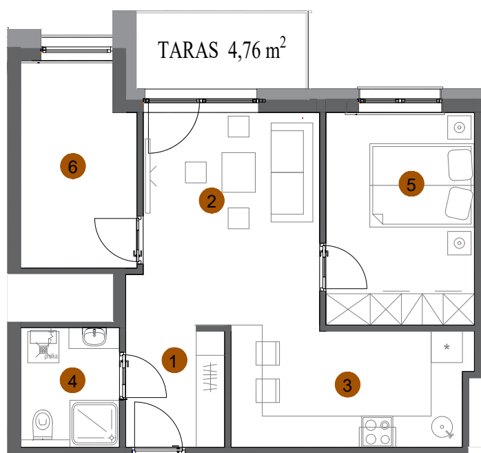
RZUT MIESZKANIA
