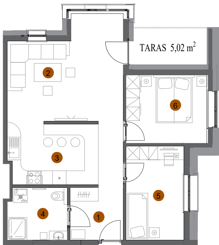
RZUT MIESZKANIA
